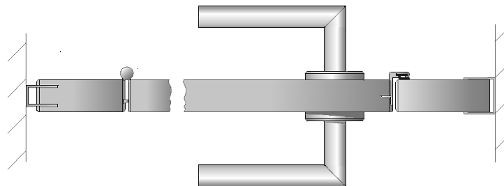
2 Vista planimetrica frontale con porta con cerniera 180°
