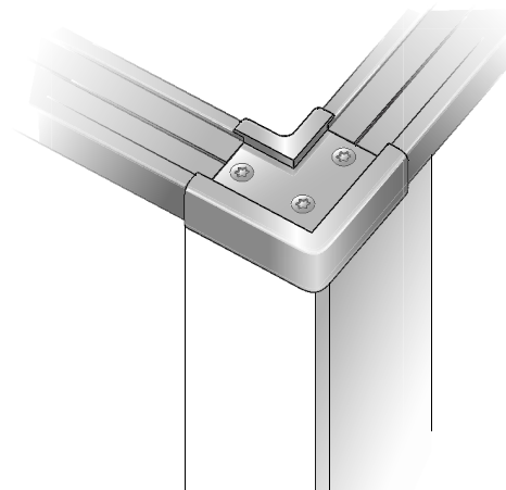
4 Raccordo angolare
