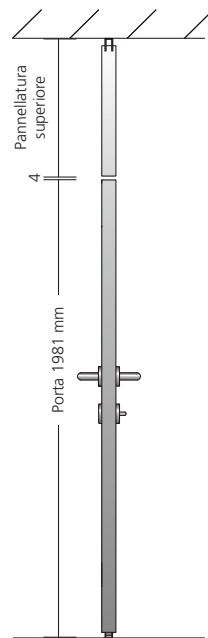
6 Sezione verticale
