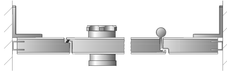
2 Vista planimetrica frontale con porta con cerniera fino a 180° (staffe di fissaggio in alluminio all'interno della cabina)
