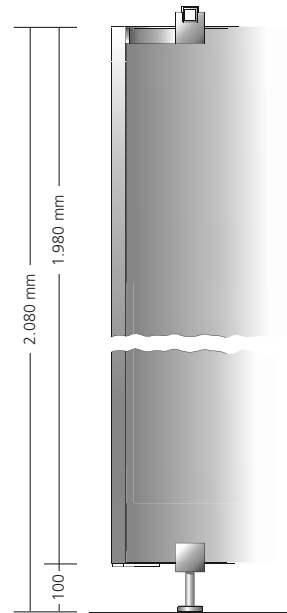
Sezione verticale
