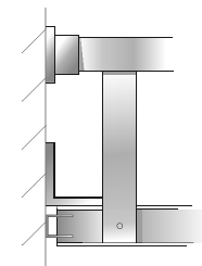
5 Fissaggio profilo superiore a parete
