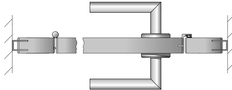
2 Schnitt Kabinenfront mit Drückergarnitur
