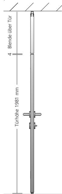
6 Höhenschnitt Front
